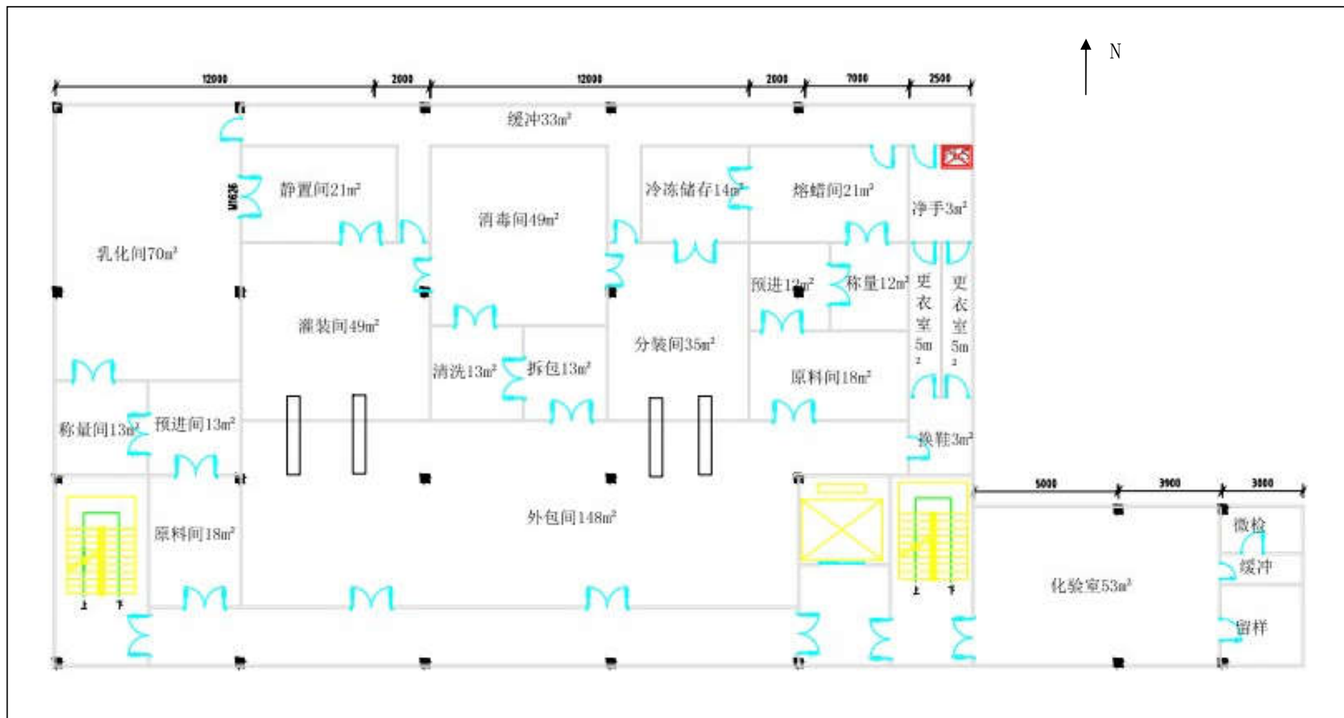
附图 4 厂房 2 层平面布置图
