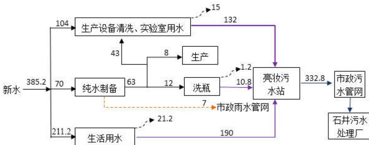
图 1 本项目用水平衡图 (单位: m 3 /a)
