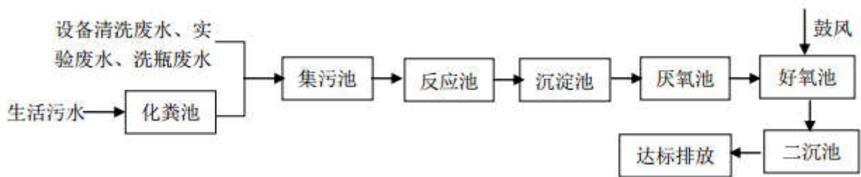
图 2 废水处理工艺流程图
